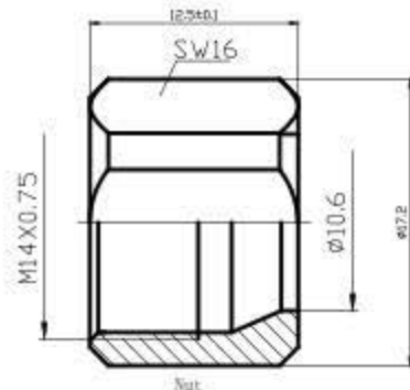
Nut
